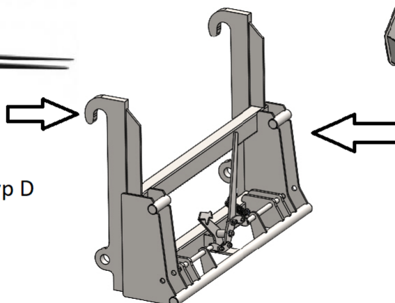
Adapter Euro mocowanie JCB typ D
