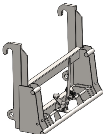
Adapter Euro mocowanie JCB typ D
