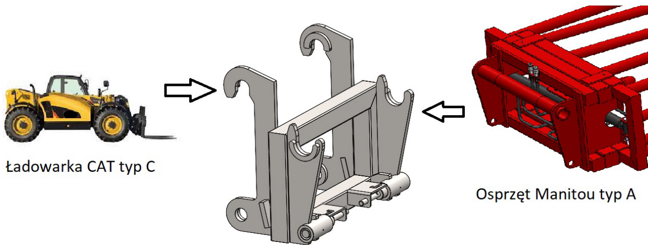
Adapter Manitou typ A mocowanie CAT typ C
